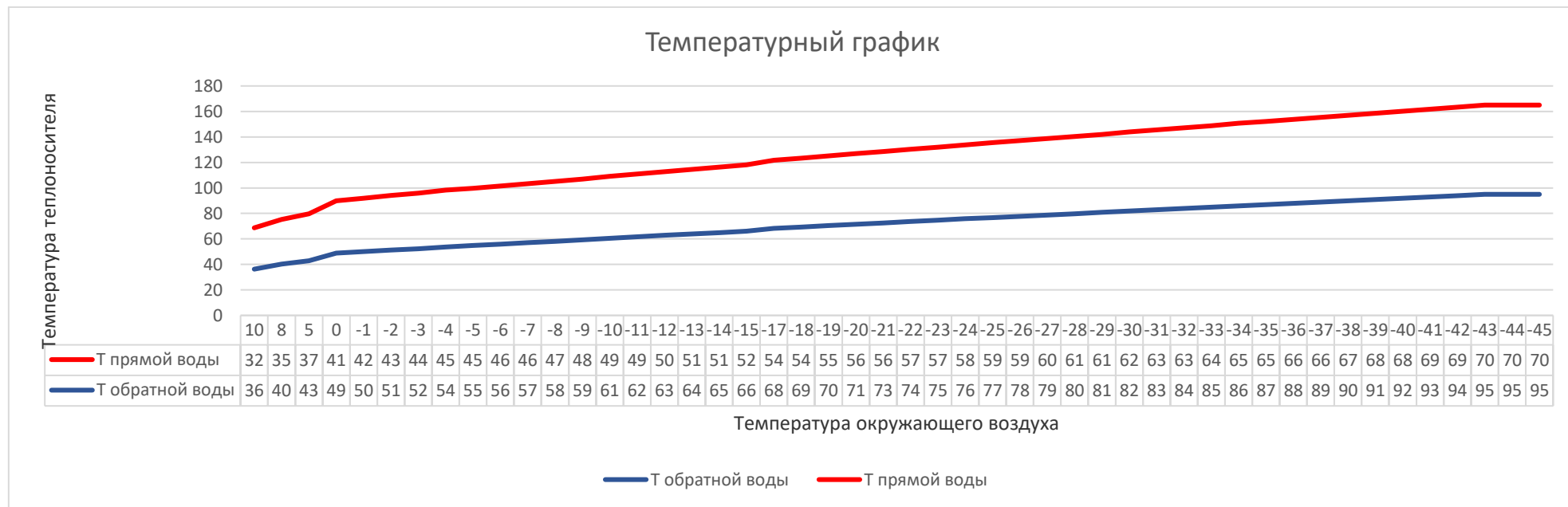
Рисунок 2 - Температурный график котельных МУП «СЖКХ»
